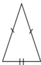
Isósceles As medidas dos dois lados são iguais.
