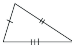
Escaleno As medidas de seus lados são diferentes.
