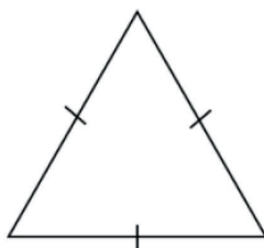
Equilátero As medidas de seus lados são iguais.
